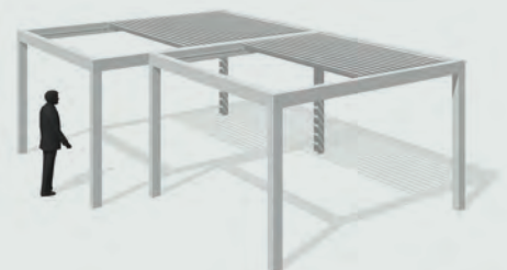
Struttura realizzata accoppiando due moduli con profondità diverse Structure made with two modules of different depth
